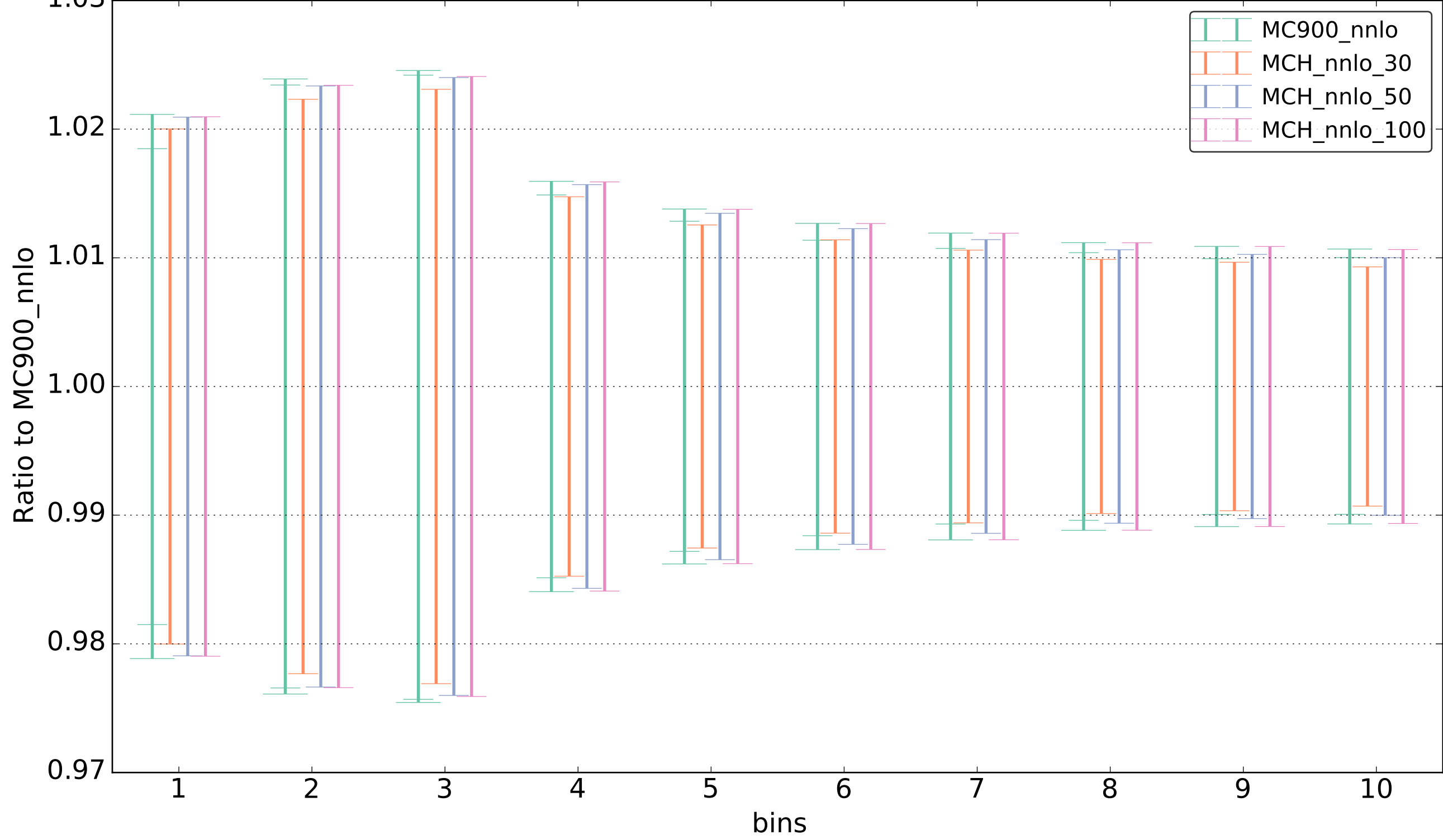
z_lppt_13tev(NLO)
