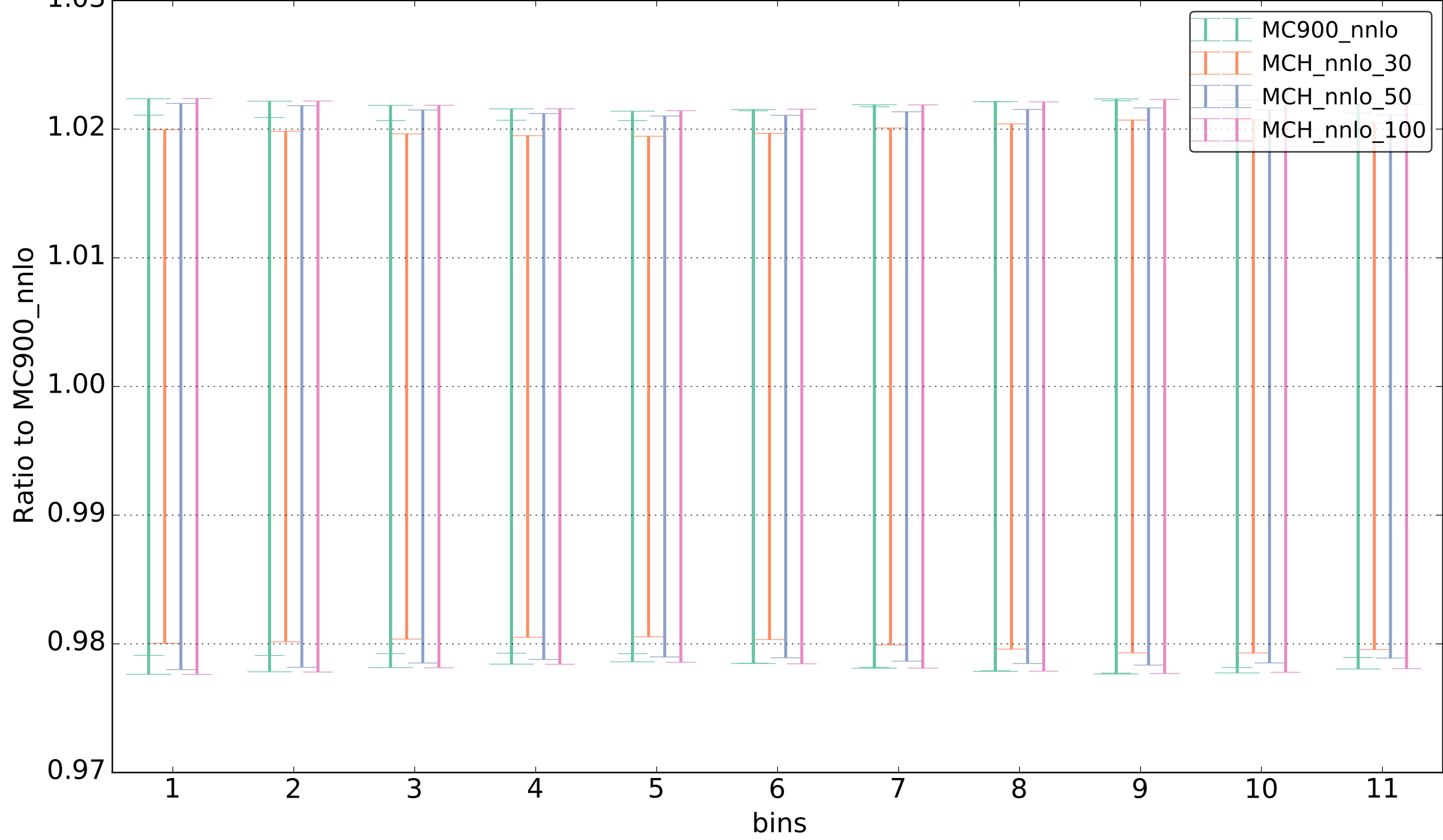
ATLAS-arXiv:1109.5141-Wminus_eta3(NLO)
