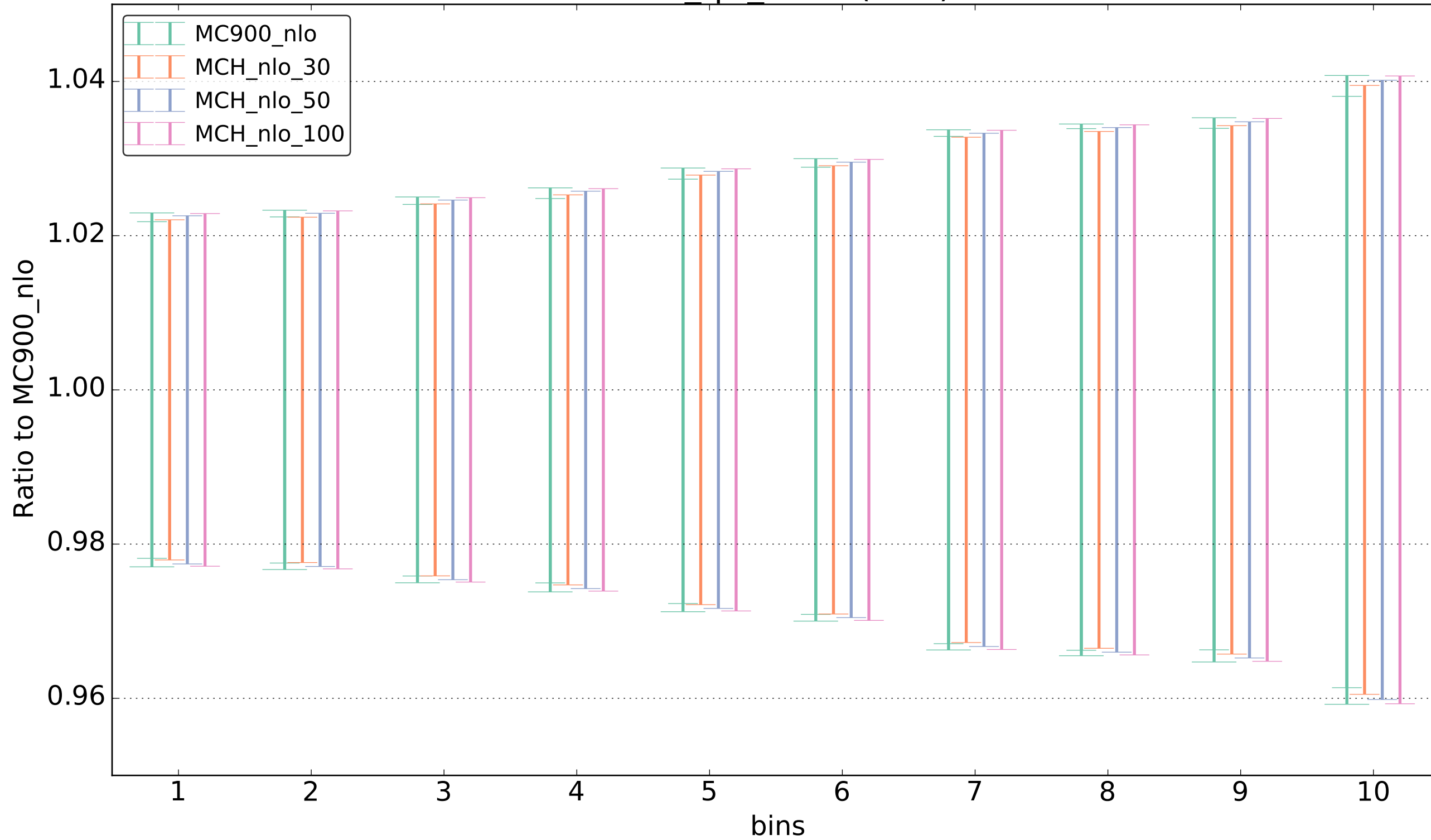
ttbar_tpt_13tev(NLO)
