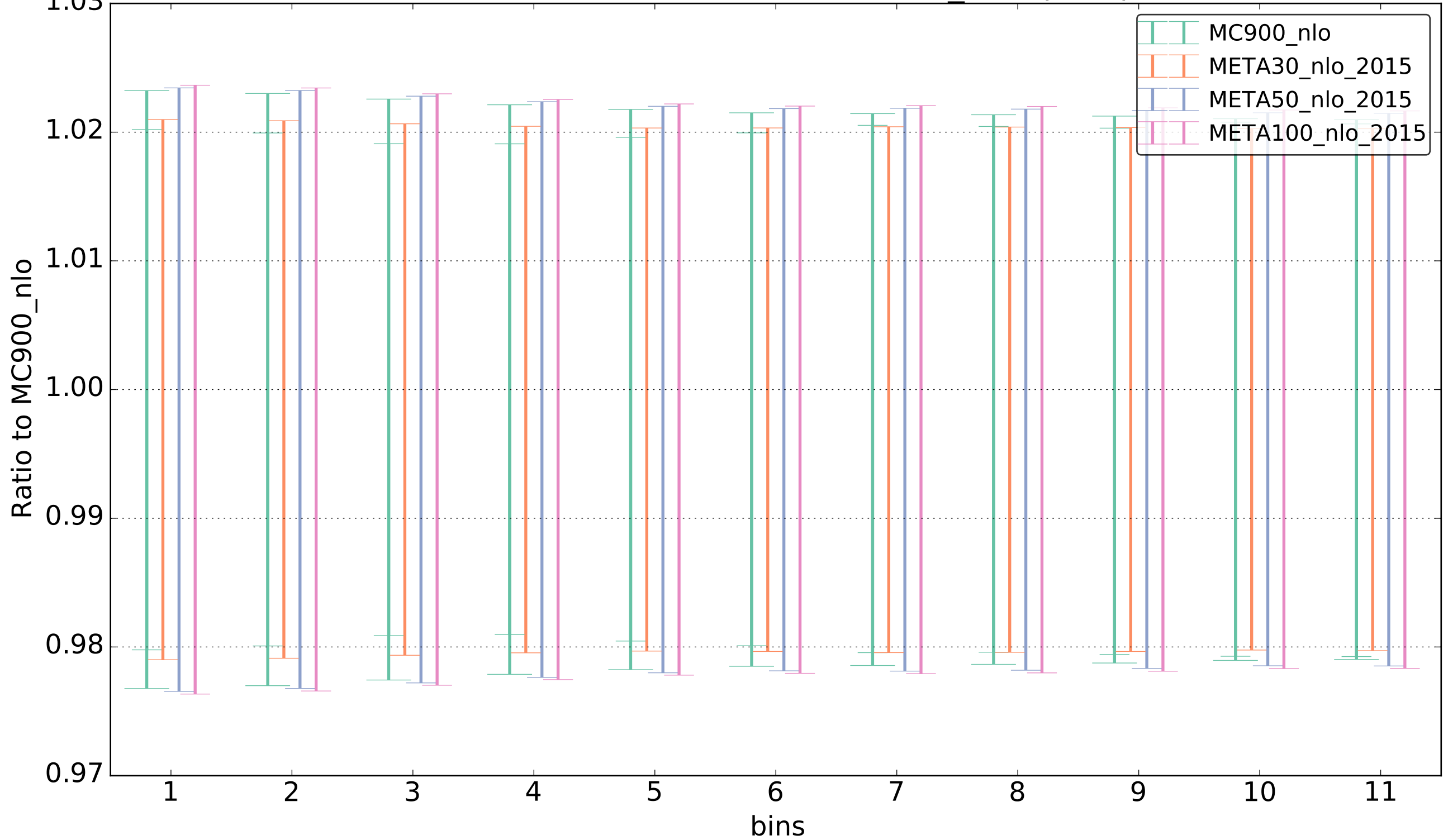
ATLAS-arXiv1109.5141-Wminus_eta3(NLO)
