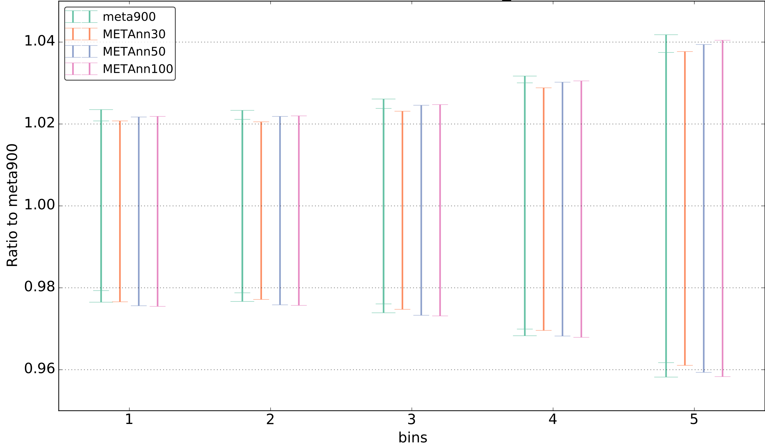
LHCb-arXiv-1204.1620-Wminus_eta3(NLO)
