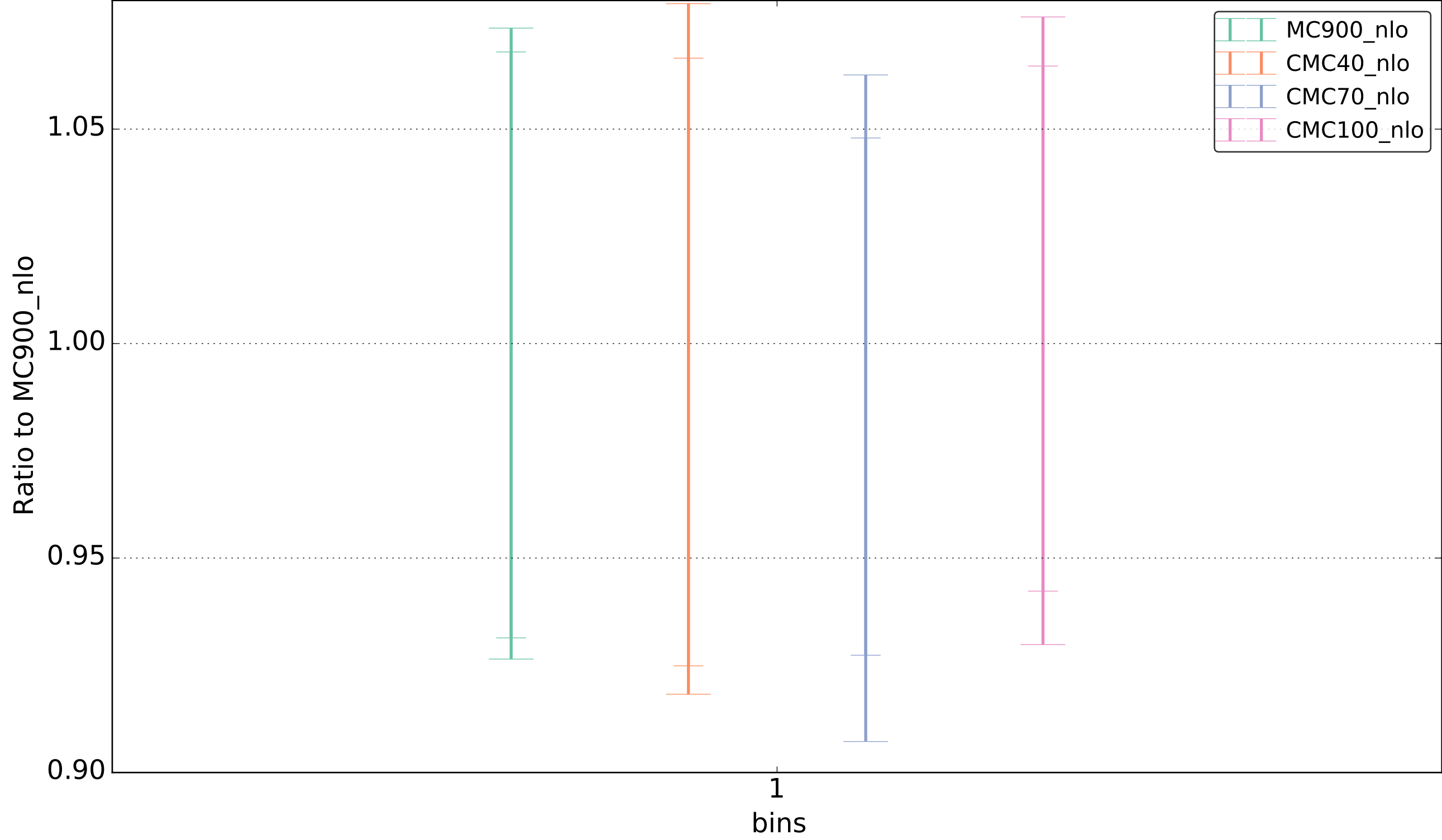
ttbar-xsectot-teva(NLO)
